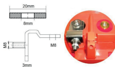
M8 Gewindebolzen Front Terminal
