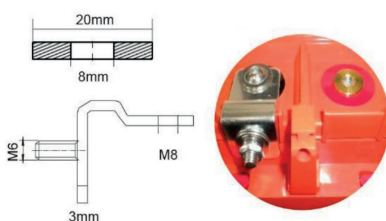
M6 Gewindebolzen Front Terminal
